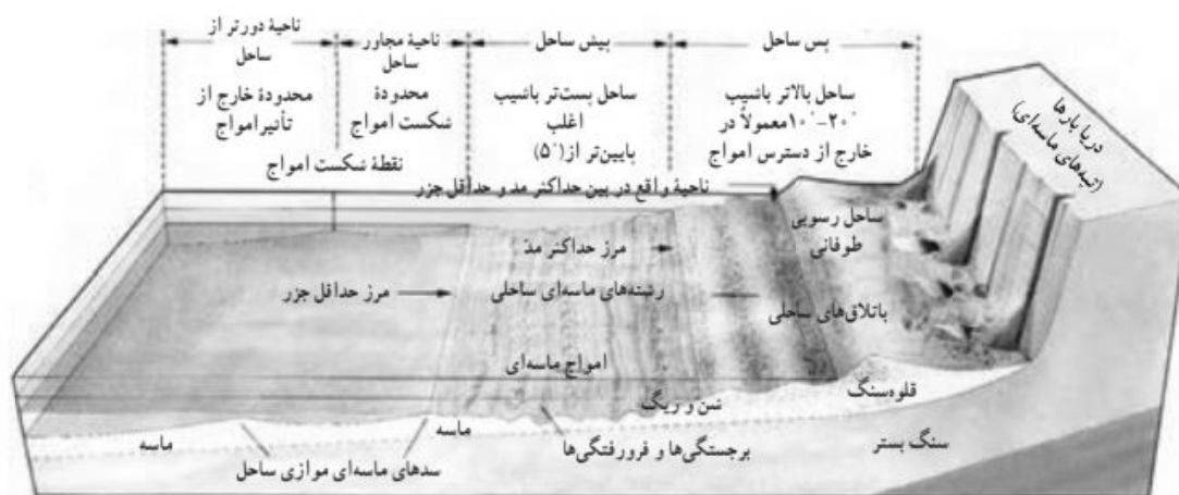
شکل ۴ - محدوده تحت تأثیر امواج و اشکال ناهمواری‌های ساحل رسوبی
